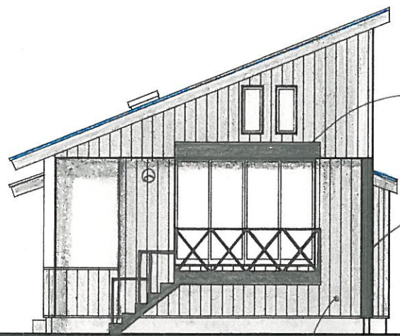
南側立面図 1 / 100
