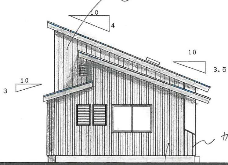
北側立面図 1 / 100
