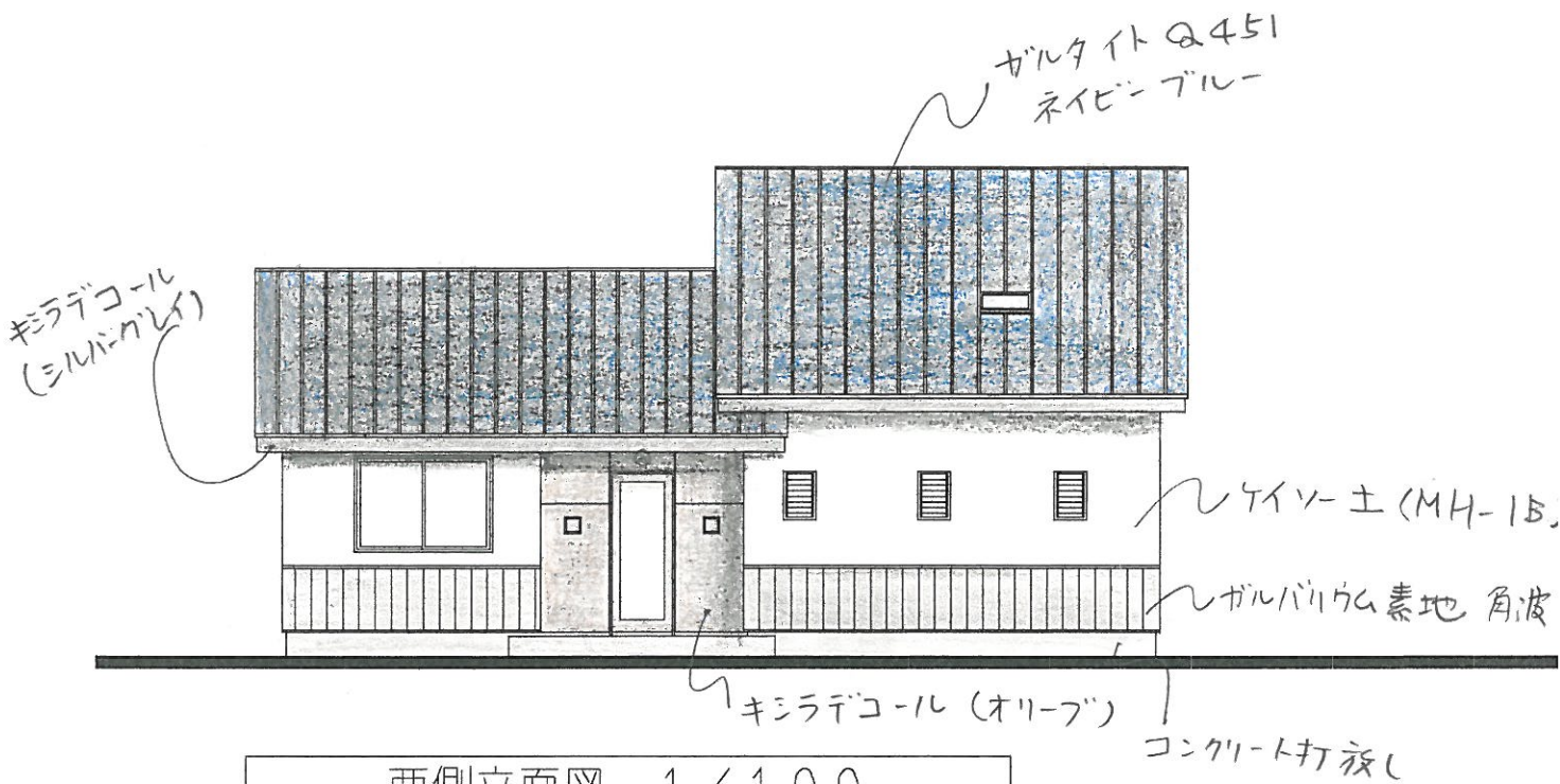
西側立面図 1 / 100
